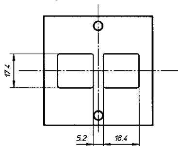
Måttritning
