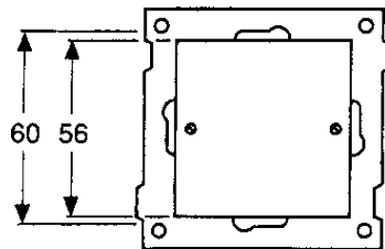
Mått ritning
