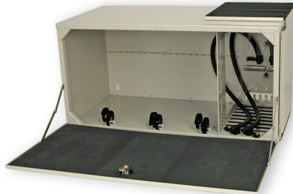
Skarvskåp T20 för fiberoptiska accessnät och volymskarvning i trunknät
